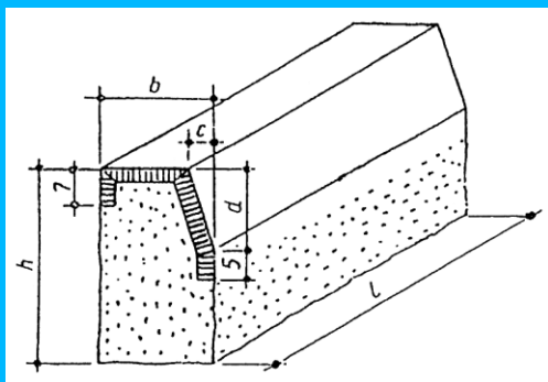
Krawężnik uliczny rodzaju A
